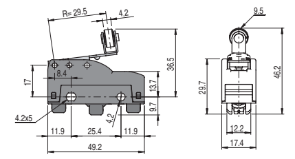
MK V11F46 → 1S+1Ö PC 1,1 mm FS 1,3 N OC 6,6 mm FR 0,9 N CD 0,1 mm FAP 6,9 N CAP 6,3 mm
