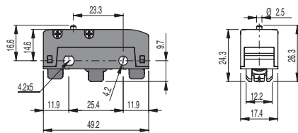
MK V11D01 1S+1Ö PC 0,5 mm FS 4 N OC 1,5 mm FR 3 N CD 0,05 mm
