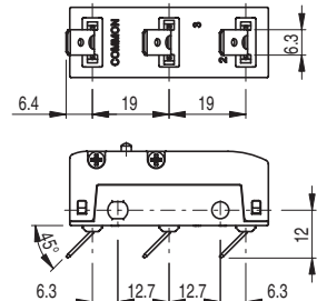
Fastonanschluß G , nach links gebo- gen (auf Anfrage)
