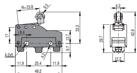
MK V11F59 → 1S+1Ö PC 0,8 mm FS 1,7 N OC 5,2 mm FR 1,3 N CD 0,08 mm FAP 8,9 N CAP 4,9 mm
