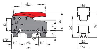
MK V11F49 → 1S+1Ö PC 1,5 mm FS 1 N OC 7,5 mm FR 0,7 N CD 0,2 mm FAP 4,8 N CAP 9 mm
