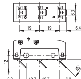
Fastonanschluß F , nach rechts gebogen
