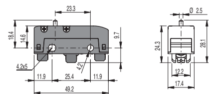
MK V11D02 1S+1Ö PC 0,5 mm FS 4 N OC 2 mm FR 3 N CD 0,05 mm
