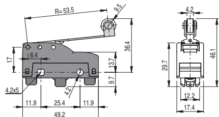
MK V11F40 1S+1Ö PC 2,4 mm FS 0,85 N OC 10,4 mm FR 0,65 N CD 0,25 mm
