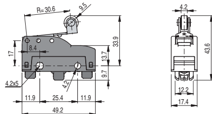
MK V11F45 → 1S+1Ö PC 1,1 mm FS 1,3 N OC 6,6 mm FR 0,9 N CD 0,1 mm FAP 6,9 N CAP 6,3 mm
