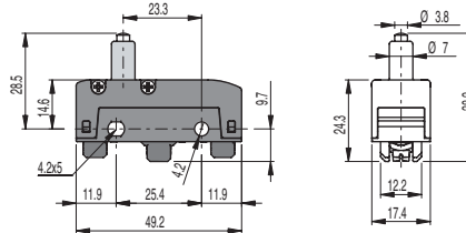
MK V11D04 1S+1Ö PC 0,5 mm FS 4 N OC 2 mm FR 3 N CD 0,05 mm
