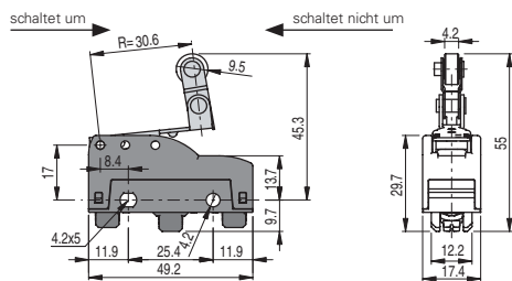
MK V11F47 → 1S+1Ö PC 1,1 mm FS 1,3 N OC 5,6 mm FR 0,9 N CD 0,1 mm FAP 6,9 N CAP 6,3 mm
