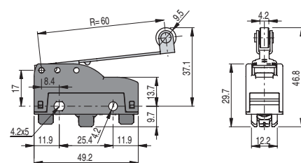
MK V11F53 1S+1Ö PC 2,5 mm FS 0,7 N OC 11,5 mm FR 0,6 N CD 0,3 mm
