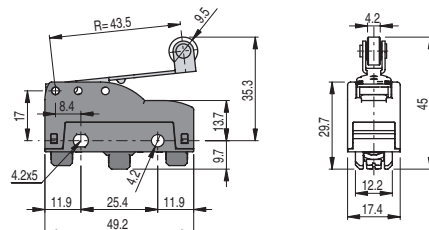
MK V11F42 → 1S+1Ö PC 1,6 mm FS 1 N OC 8,4 mm FR 0,7 N CD 0,2 mm FAP 4,9 N CAP 9 mm
